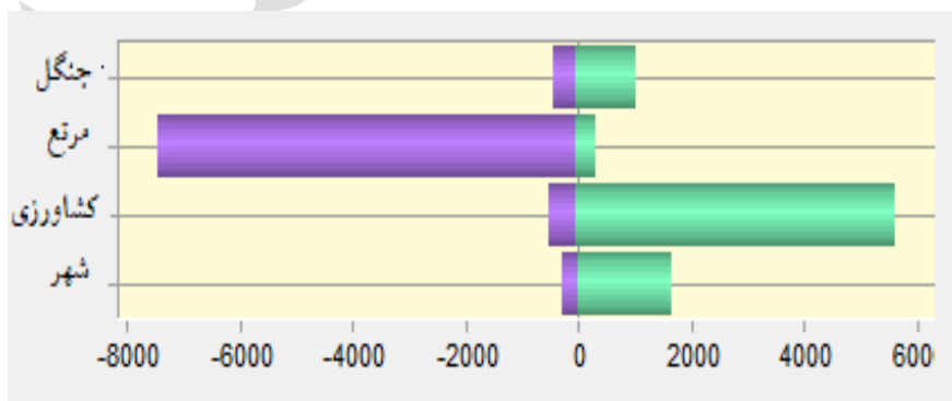
شکل ۹. تغییرات کاربری اراضی کلان شهر اراک بین سال‌های ۱۹۷۶ تا ۱۹۹۶
