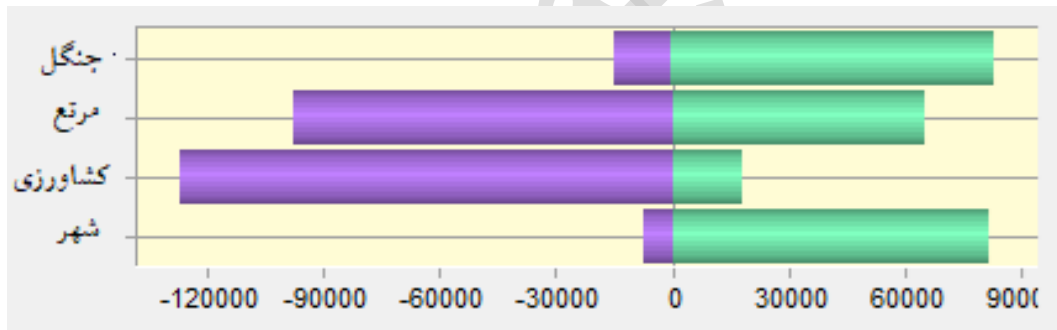
شکل ۱۰. تغییرات کاربری اراضی کلان‌شهر اراک بین سال‌های ۱۹۹۶ تا ۲۰۲۴
