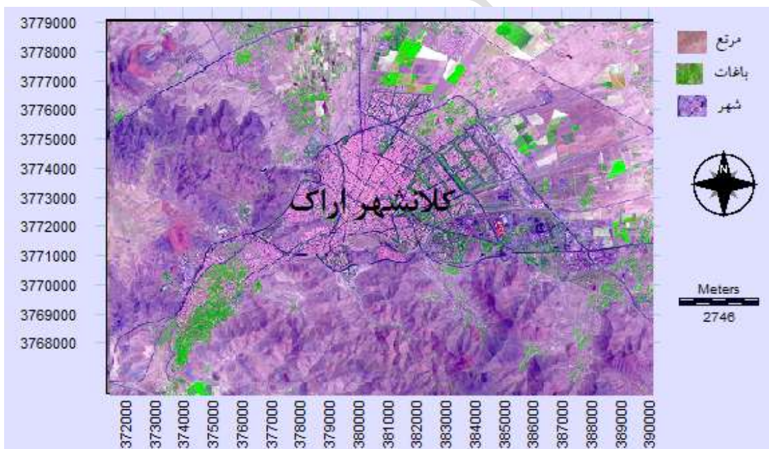
شکل ۳. تصاویر ماهواره ای لندست سال ۲۰۲۴
