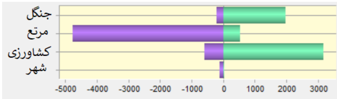
شکل ۱۱. تغییرات کاربری اراضی کلان‌شهر اراک بین سال‌های ۱۹۷۶ تا ۲۰۲۴
