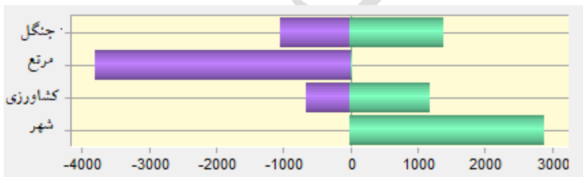
شکل ۱۳. تغییرات کاربری اراضی کلان‌شهر اراک بین سال‌های ۲۰۲۴ تا ۲۰۴۰
