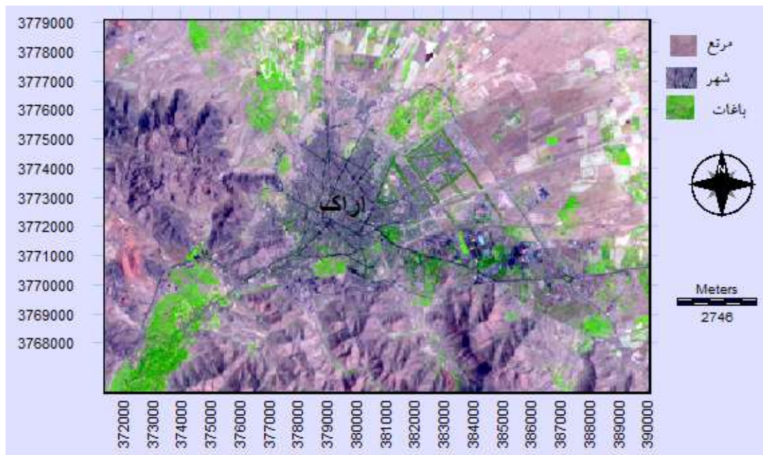
شکل ۲. تصاویر ماهواره ای لندست سال ۱۹۹۶
