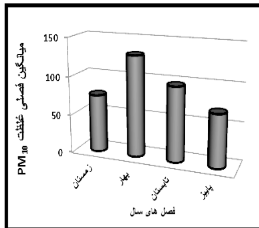
شکل ۳. میانگین فصلی ذرات معلق طی سال‌های ۲۰۰۸-۲۰۱۲
