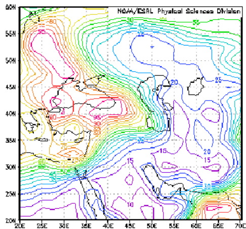
شکل ۱۷. نقشه رطوبت نسبی سطح زمین در روز ۲۴ ژوئن ۲۰۱۰ ( http://www.esrl.noaa.gov )
