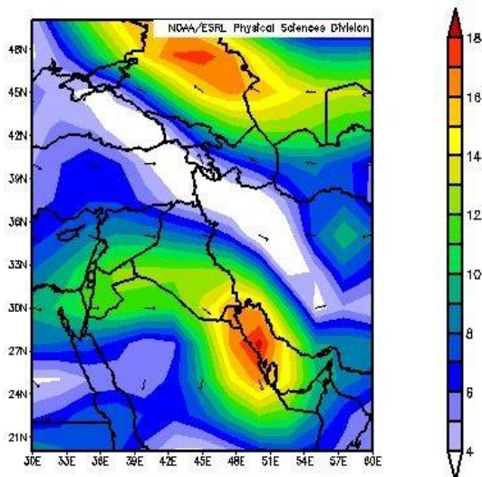
شکل ۱۸. نقشه جهت و سرعت باد در سطح ۸۵۰ هکتوپاسکال، روز ۲۴ ژوئن ۲۰۱۰ ( http://www.esrl.noaa.gov )
