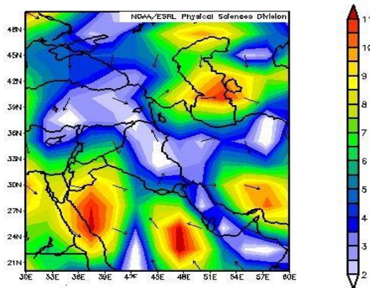
شکل ۲۷. نقشه جهت و سرعت باد در سطح ۸۵۰ هکتوپاسکال، روز ۱۴ می ۲۰۱۱ ( http://www.esrl.noaa.gov )
