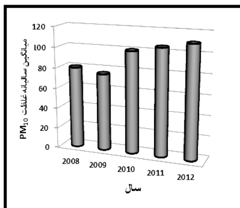
شکل ۲. میانگین سالیانه ذرات معلق طی سال‌های ۲۰۰۸-۲۰۱۲
