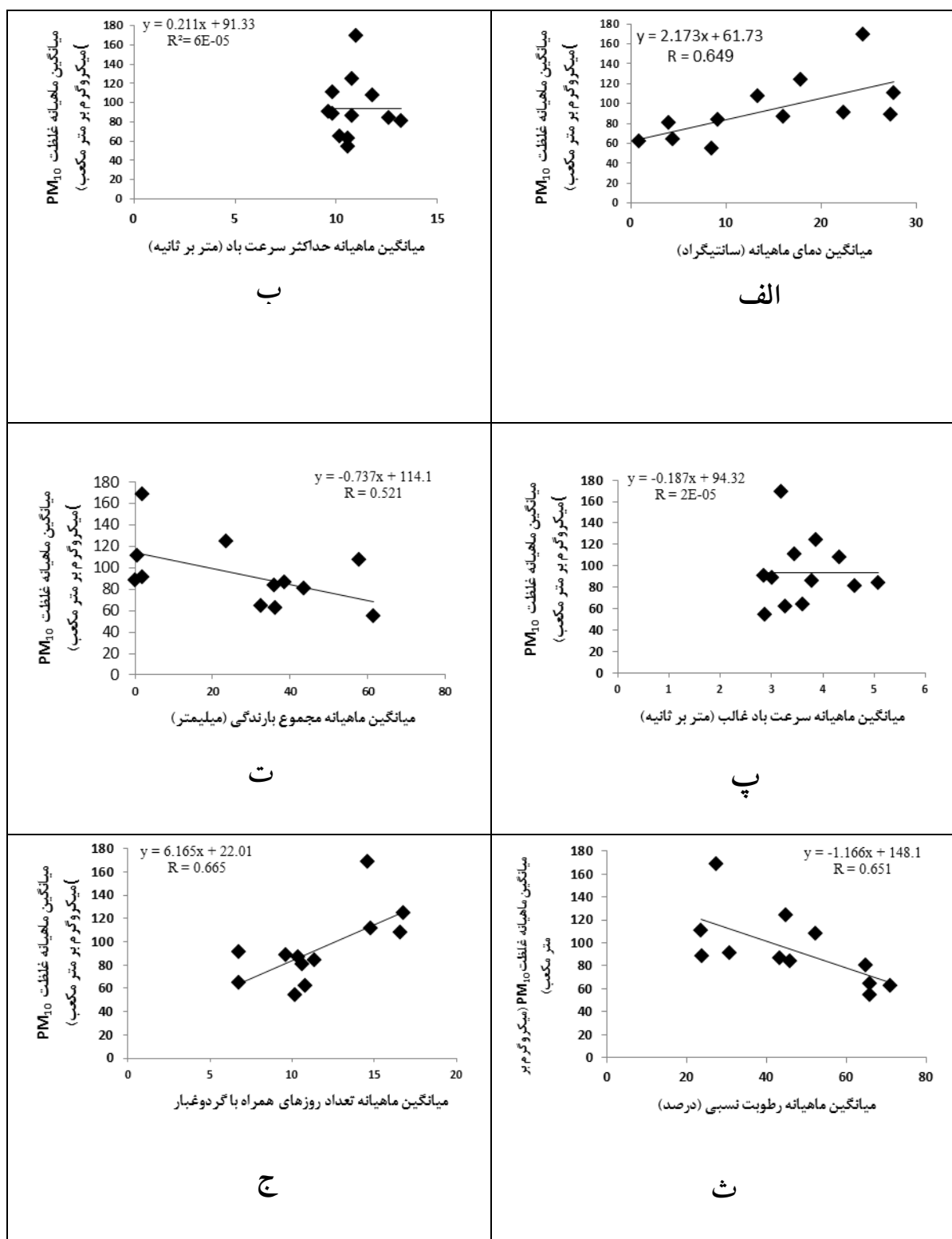
شکل ۵. رابطه رگرسیونی بین عناصر هواشناسی محلی و غلظت ذرات معلق طی سالهای ۲۰۰۸-۲۰۱۲
