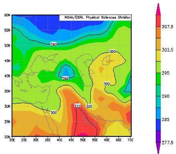
شکل ۸. نقشه خطوط هم دمای سطح زمین در روز ۵ جولای ۲۰۰۹ ( http://www.esrl.noaa.gov )
