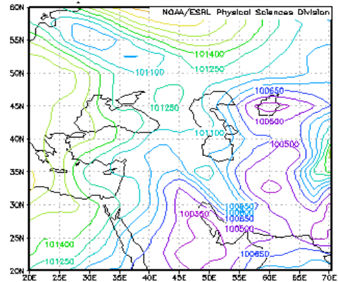
شکل ۲۴. الگوی آرایش فشار در نقشه تراز دریا،
