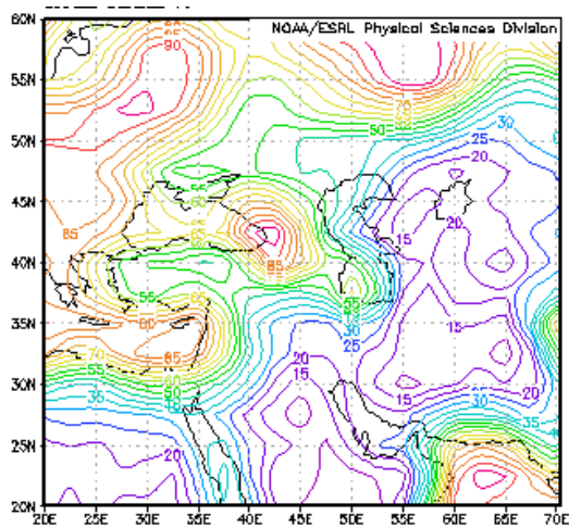
شکل ۹. نقشه رطوبت نسبی سطح زمین در روز ۵ جولای ۲۰۰۹ ( http://www.esrl.noaa.gov )
