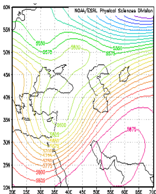
شکل ۲۳. الگوی آرایش ارتفاع تراز ۵۰۰ هکتوپاسکال، روز ۱۴ می ۲۰۱۱ ( http://www.esrl.noaa.gov )
