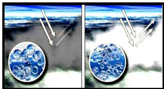
شکل ۱. تأثیر ذرات گرد و غبار بر تعداد و اندازه قطرات ابر: هوای با گرد و غبار (سمت راست) و هوای بدون گرد و غبار (سمت چپ). منبع: (Ismaili, 2006: 9)
