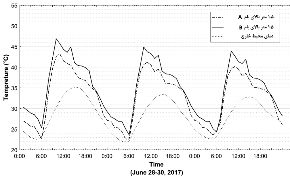
شکل ۱۰. مقایسه دمای هوا در ارتفاع ۱,۵ متری از سطح بام‌های A و B (۲۸ تا ۳۰ ماه جون)
