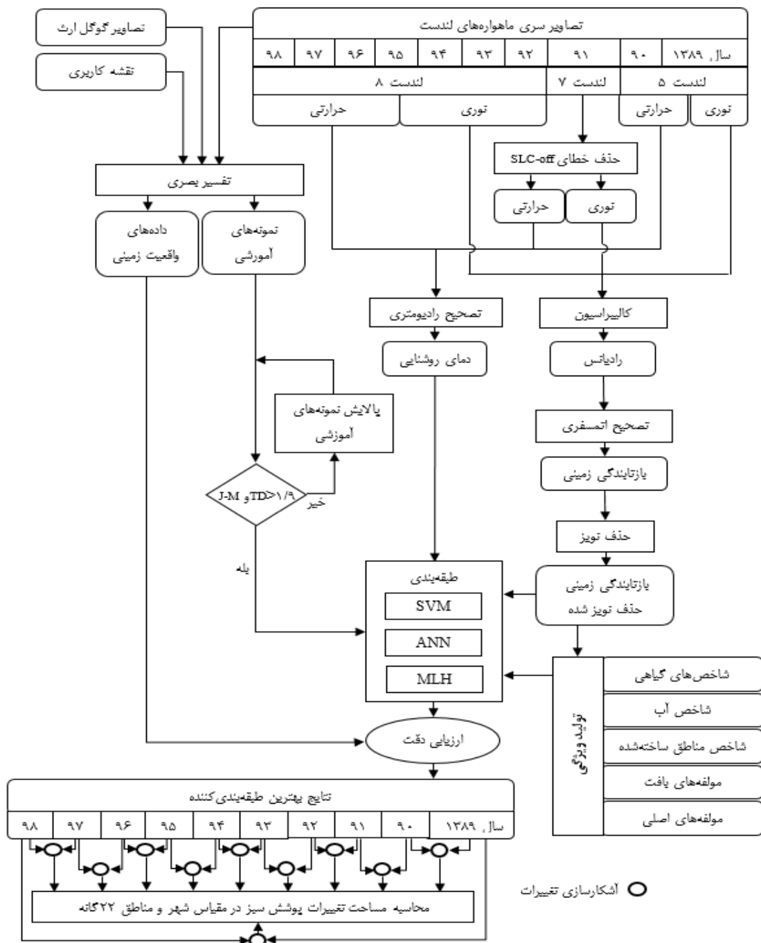
شکل ۱. فلوچارت فرآیند اجرای تحقیق
