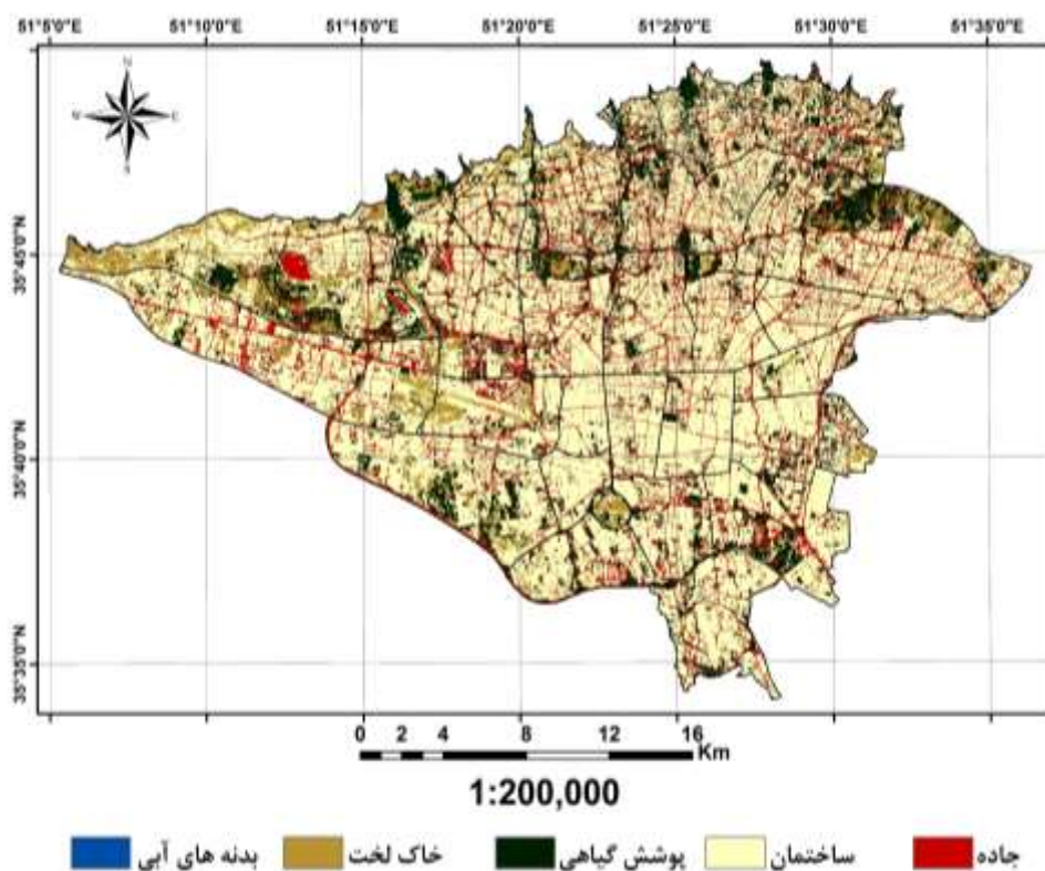
شکل ۵. ب. نقشه طبقه‌بندی شده به روش شبکه عصبی مصنوعی سال ۱۳۹۸
