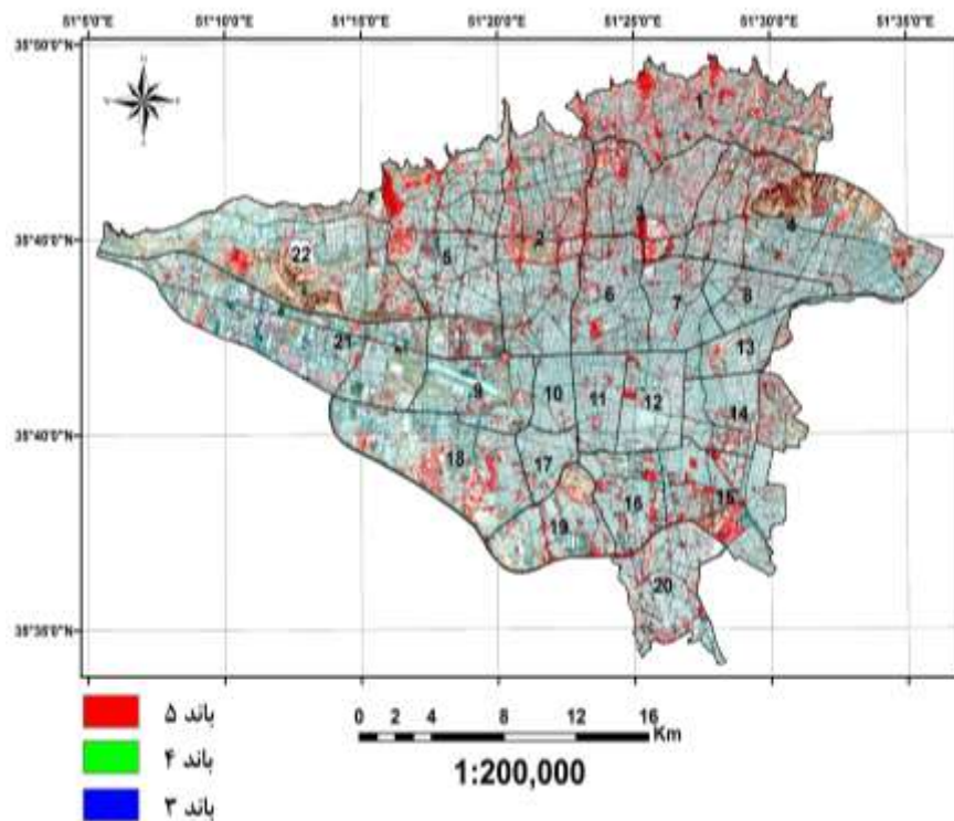
شکل ۳. تصویر ترکیب رنگی کاذب مادون قرمز تصویر بازتابندگی زمینی پس از حذف نویز سال ۱۳۹۸
