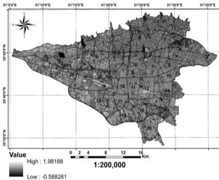
شکل ۴. الف. تصویر مؤلفه اصلی اول سال ۱۳۹۸
