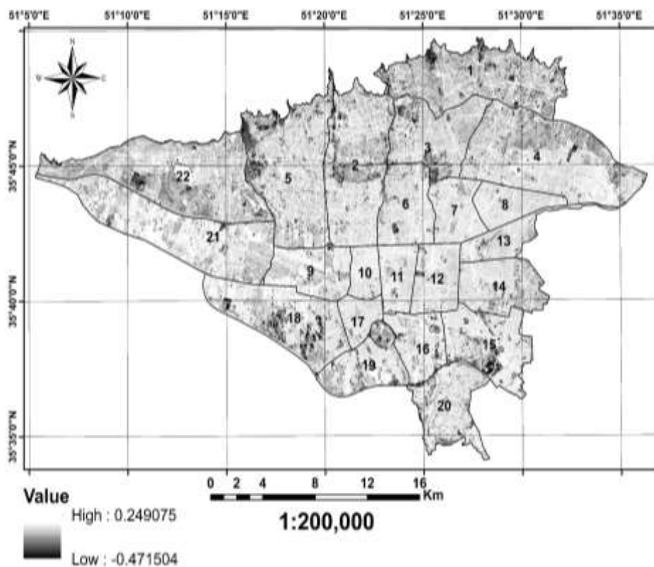
شکل ۴. ب. تصویر مؤلفه‌های اصلی دوم
