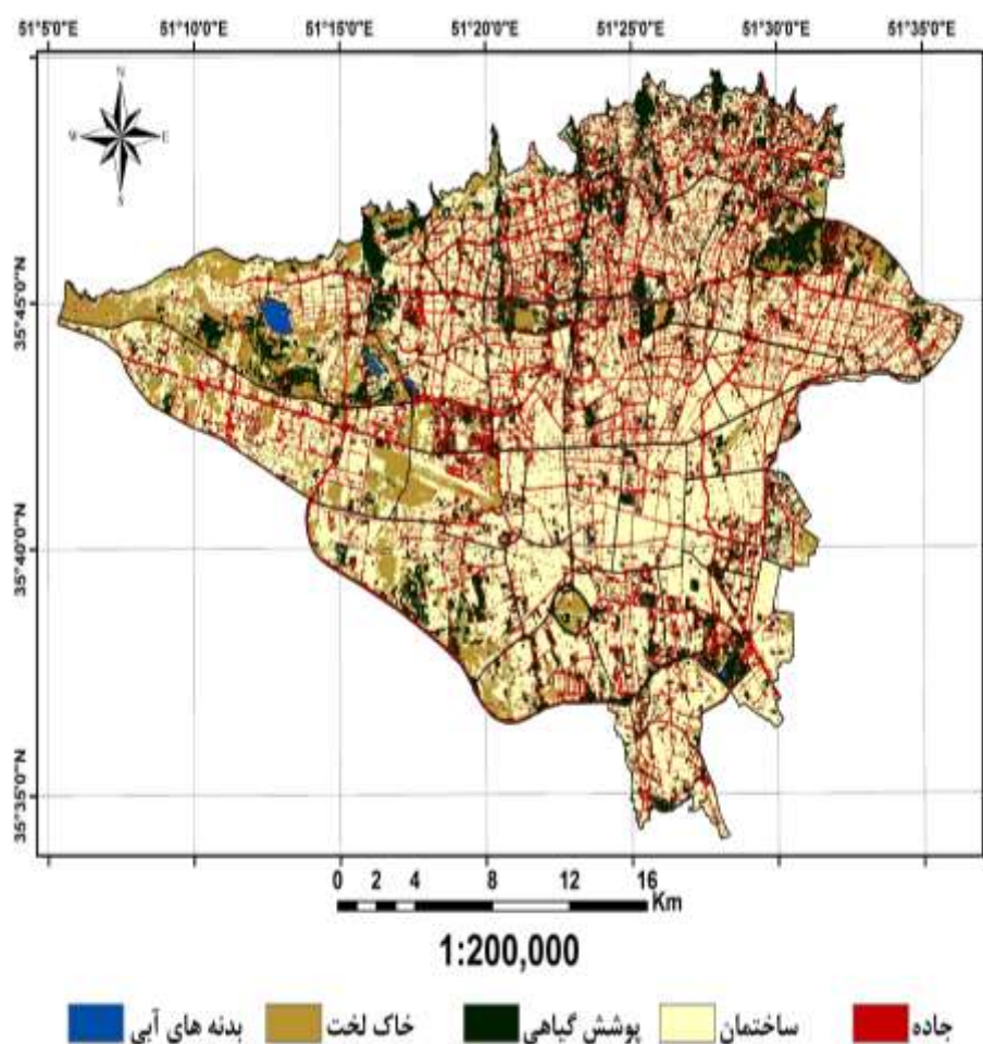
شکل ۵. الف. نقشه طبقه‌بندی شده به روش ماشین بردار پشتیبان سال ۱۳۹۸
