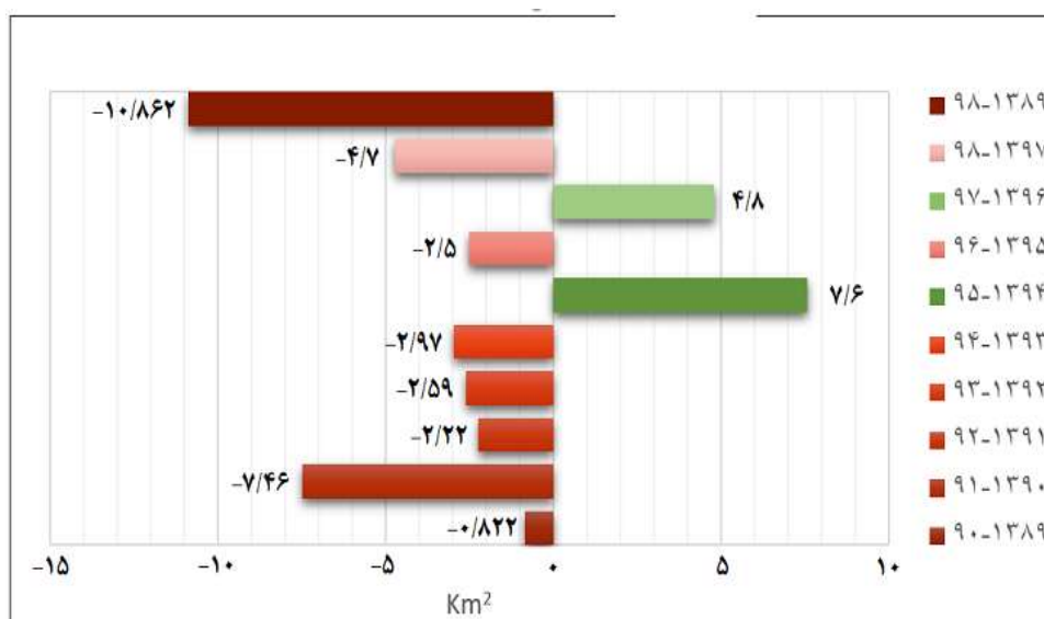
شکل ۶. تغییرات سالانه و ده‌ساله پوشش سبز در سطح شهر تهران
