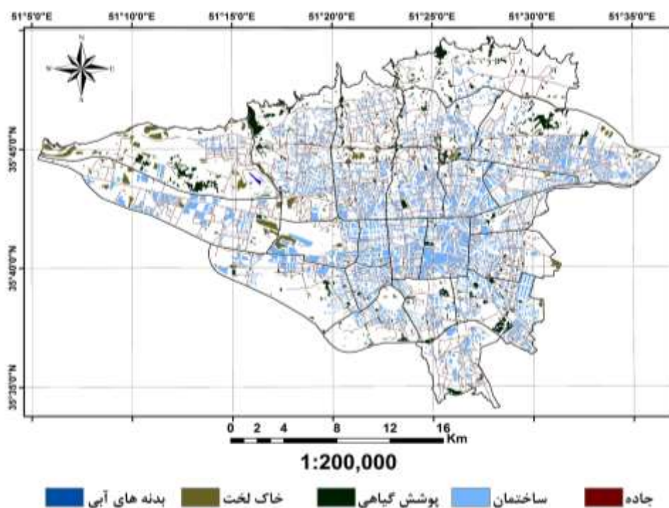
شکل ۵.۵. نقشه‌های طبقه‌بندی شده سال ۱۳۹۸ و نقشه واقعیت زمینی
