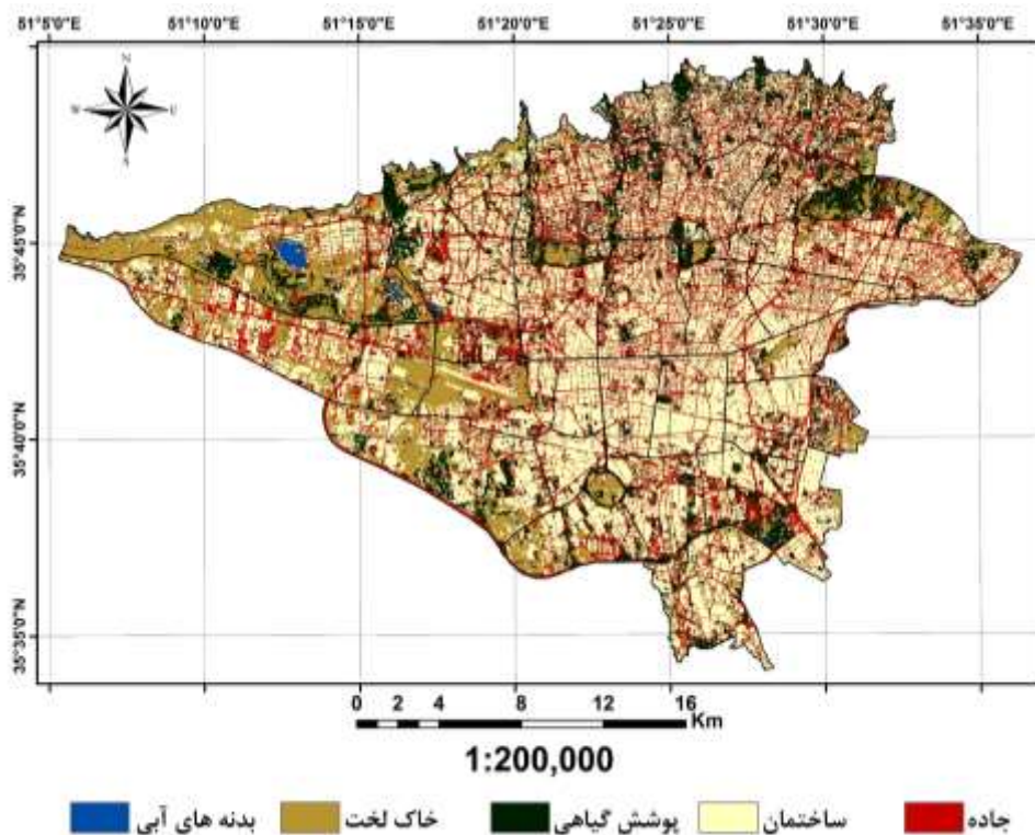
شکل ۵. ج. نقشه طبقه‌بندی شده به روش بیشترین شباهت سال ۱۳۹۸
