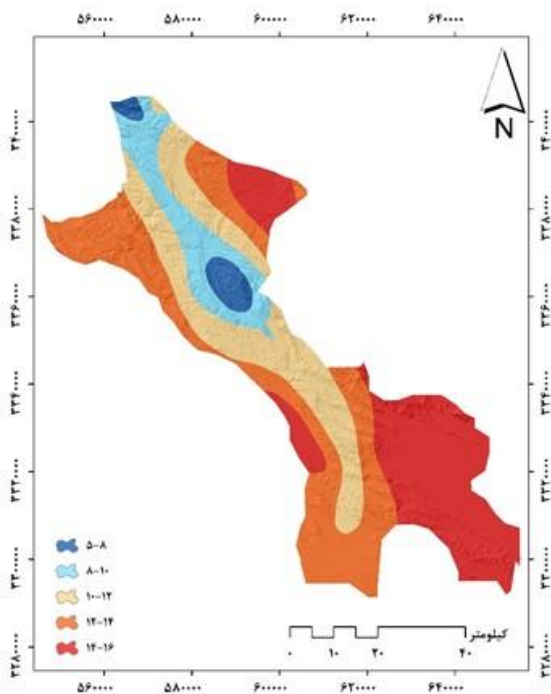
شکل ۸. نقشه دما
