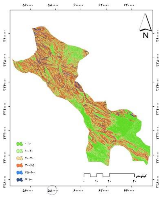
شکل ۹. نقشه شیب
