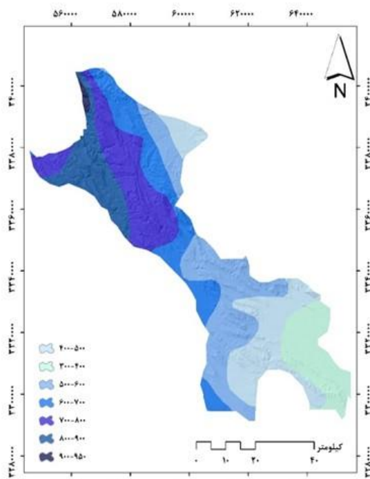
شکل ۷. نقشه بارندگی
