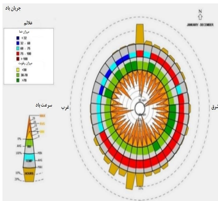
شکل ۱۰. سرعت و جهات مختلف باد به وسیله نرم‌افزار Climate Consultant از نسخه شماره ۶
