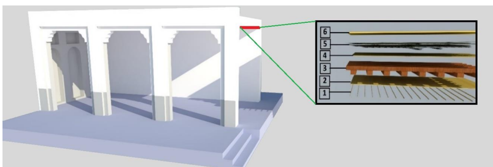
شکل ۲. مصالح به کار رفته در سقف فضاهای نیمه‌باز
