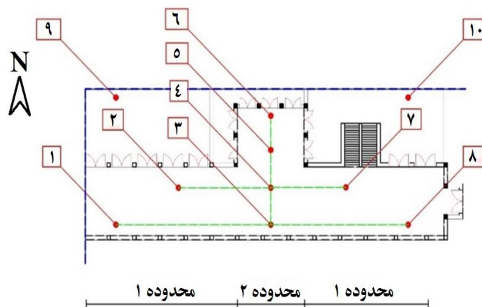
شکل ۱۵. نقاط تحلیل دما و نور در فضای نیمه‌باز و بسته بنای حاج احمد
