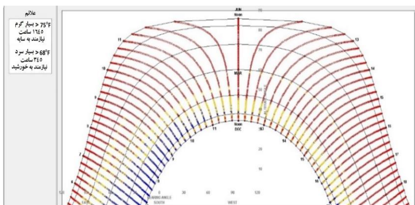
شکل ۹. سایه و آفتاب در ساعات مختلف روز در فصل گرم سال به وسیله نرم‌افزار Climate Consultant از نسخه شماره ۶
