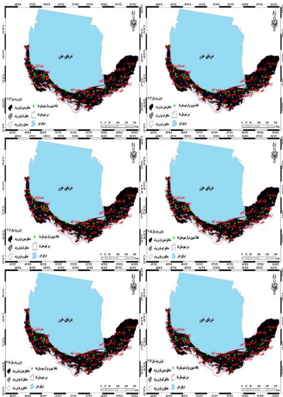
ادامه شکل ۸. نقشه تغییرات مساحت پوشش برف منطقه مورد مطالعه در دوره آماری ۲۰۱۸-۲۰۱۳
