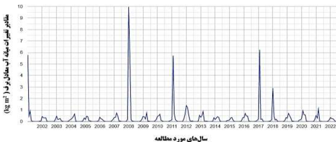
شکل ۵. نمودار تغییرات میانگین آب معادل برف در استان‌های ساحل خزری در دوره آماری ۲۰۰۱-۲۰۲۲
